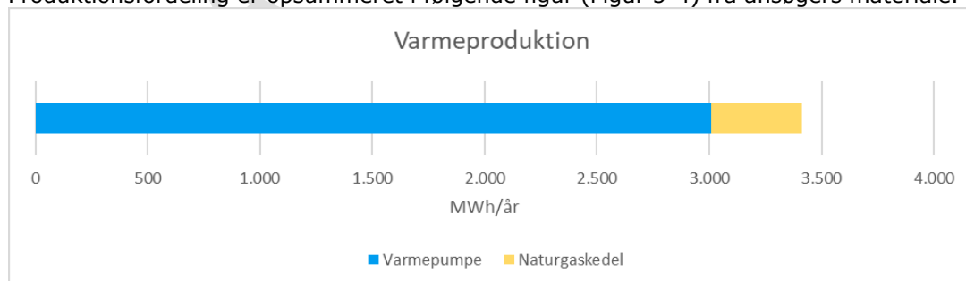
Figur 1: Samlet varmeproduktion pr. år for varmepumpen og naturgaskedlen
